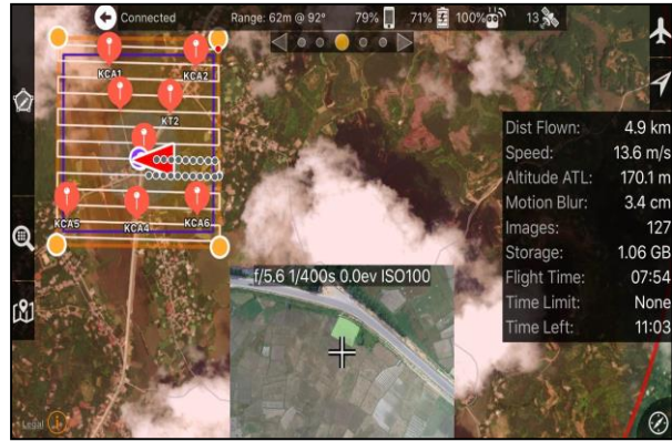
Hình 4. Sơ đồ tuyến bay được thiết kế trên phần mềm Map Pilot.
